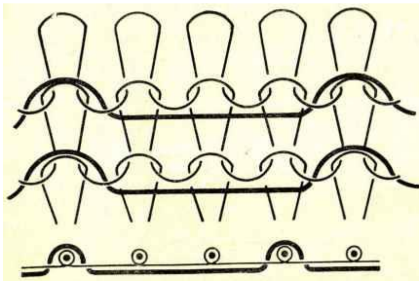
Рис. 1-1. Схема и график переплетения трико-сукно.
